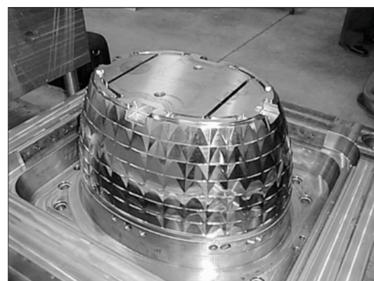
Form zur Herstellung eines Schutzglases für Straßenlaternen.
