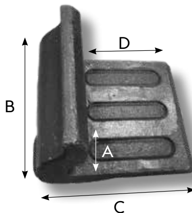
Kauhan kulmasuoja
