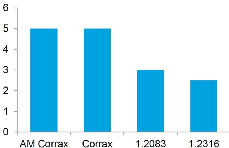
Diagrama de resistencia a la corrosión. Los valores de AM Corrax son idénticos a los del Corrax convencional.
