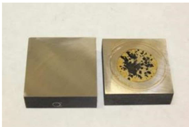
Ensayos de resistencia a la corrosión de una pieza fabricada con Uddeholm AM Corrax®
